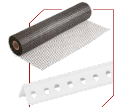
FIBRE DE VERRE 5X5 MM BAGUETTE EN PVC 2,8
