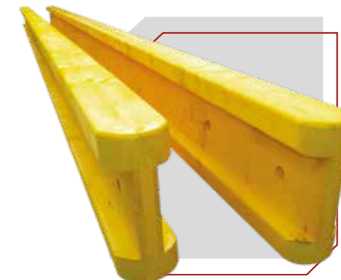
POUTRE H20 3M / 4M (L)
